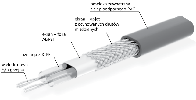
Konstrukcja przewodu grzejnego ELEKTRA VCD
