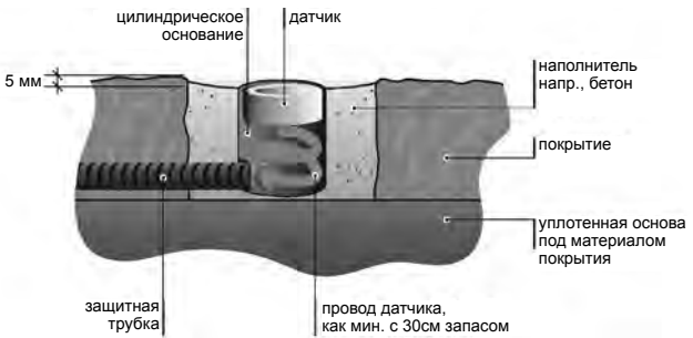
Пример монтажа датчика температуры и влажности в поверхности
